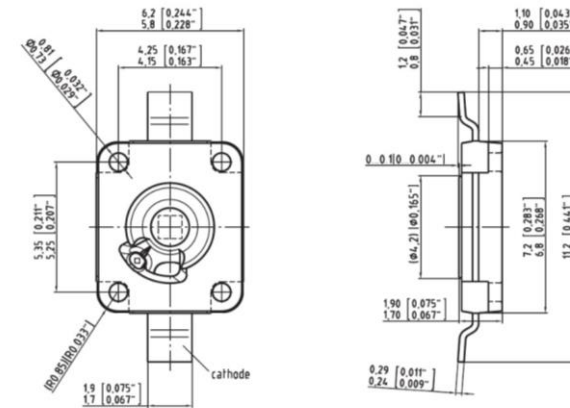
Dimensions in mm (inch). / Maße in mm (inch). Cathode mark on the bottom side / Kathodenmarkierung auf der Bauteilunterseite
