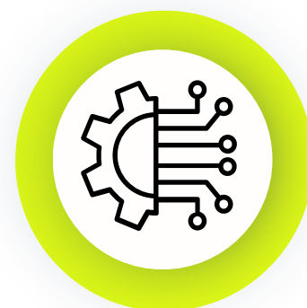
LLM
